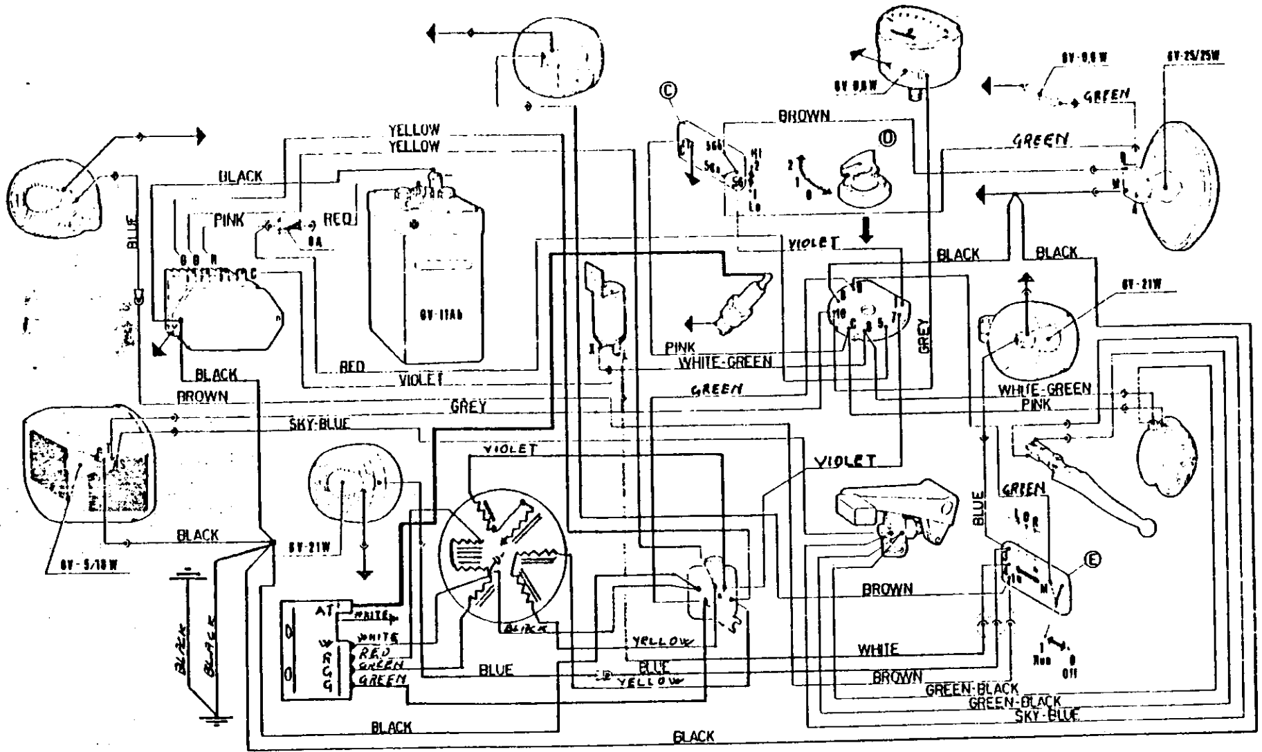
Fig. 1 - Wiring diagram
